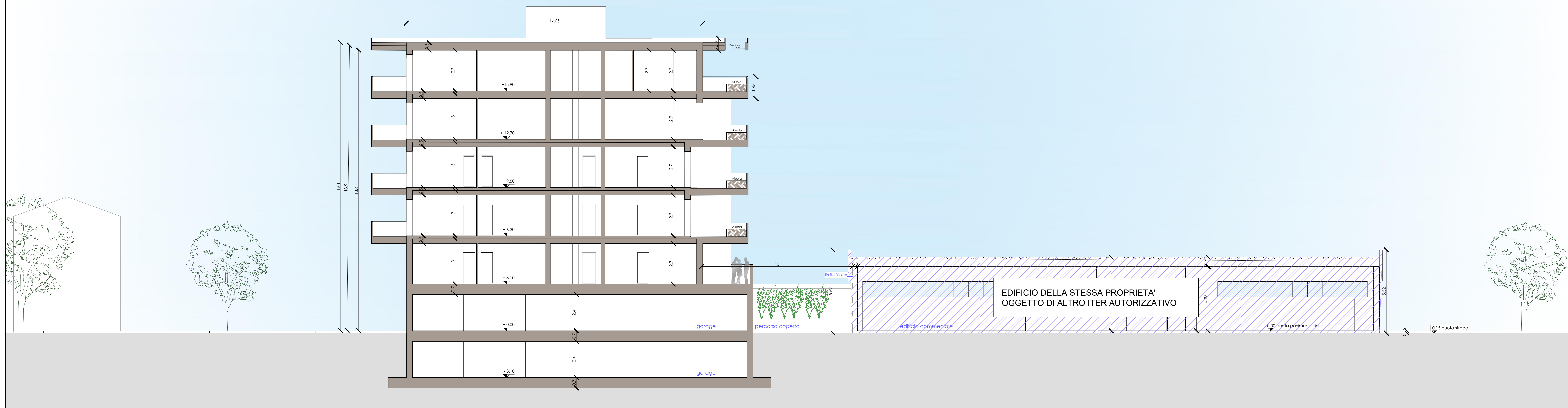
SEZIONE BB
