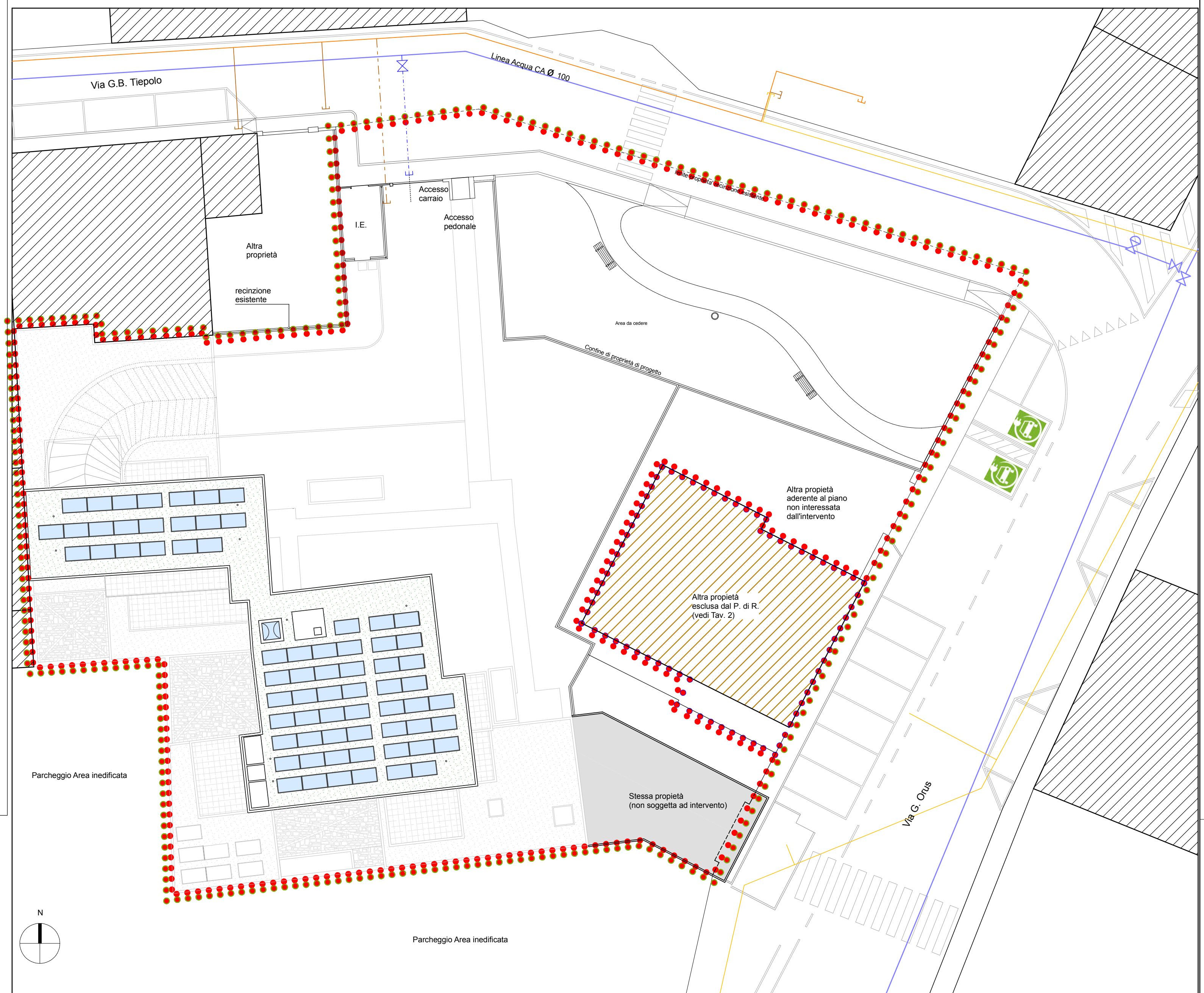
Planimetria scala 1/200
