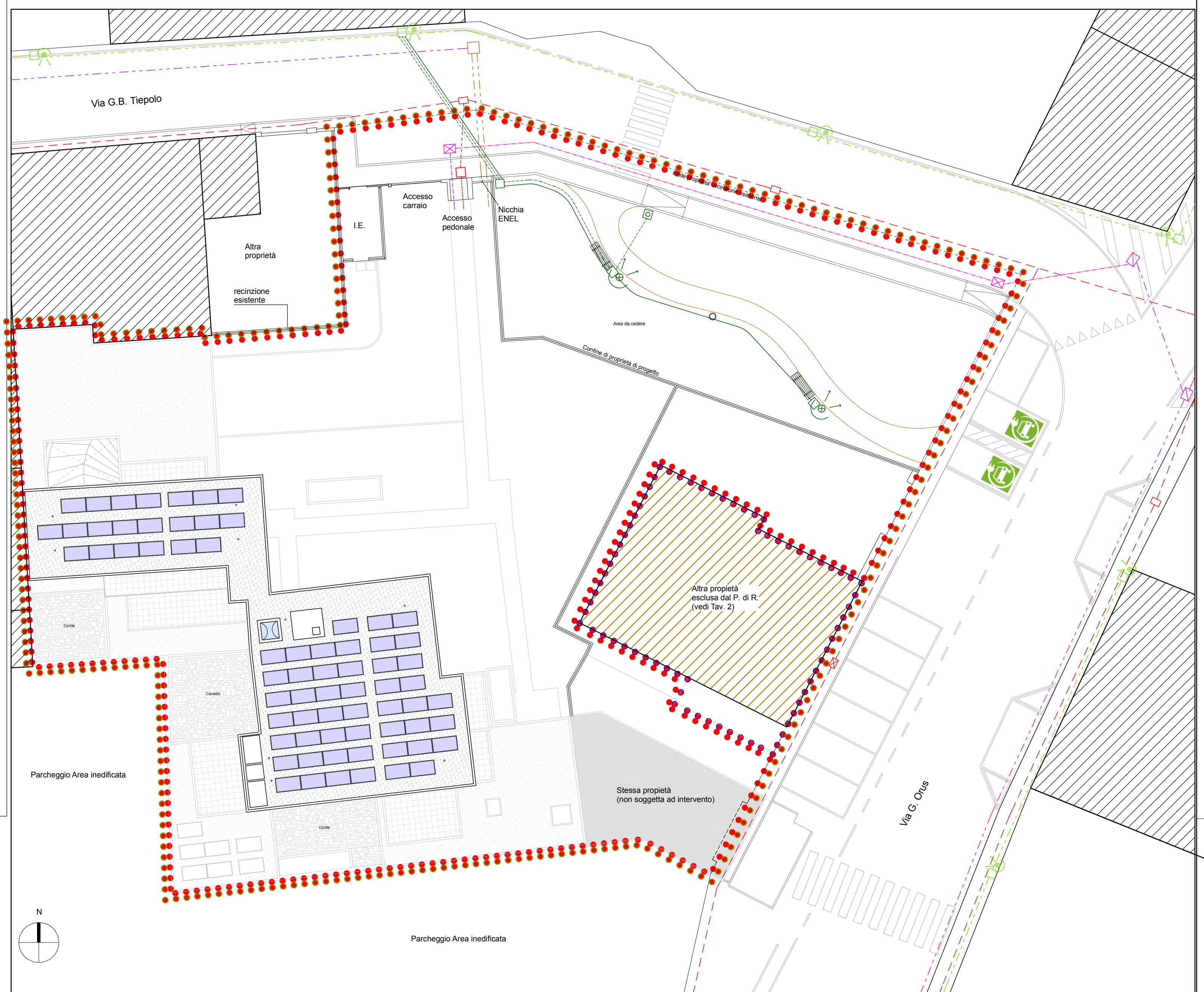
Planimetria scala 1/200
