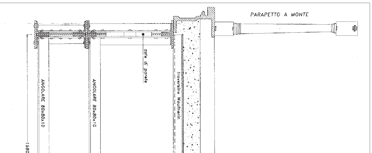
1-Particolare SEZIONE TRASVERSALE
