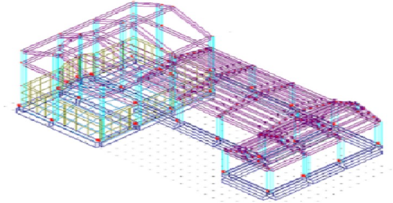
Edificio Residenziale Via Annibale da Bassano Padova
