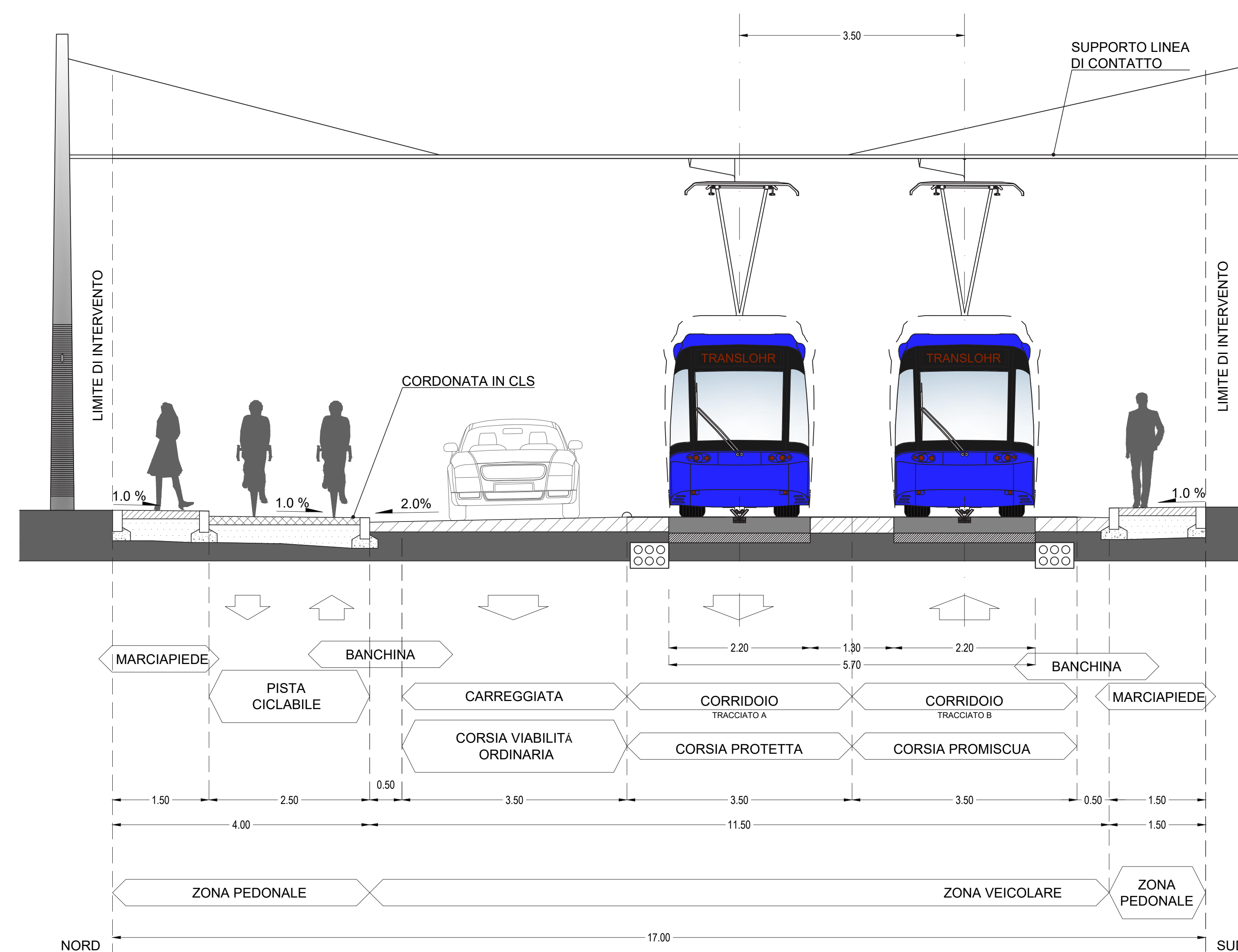
SEZIONE 10 SCALA 1:50
