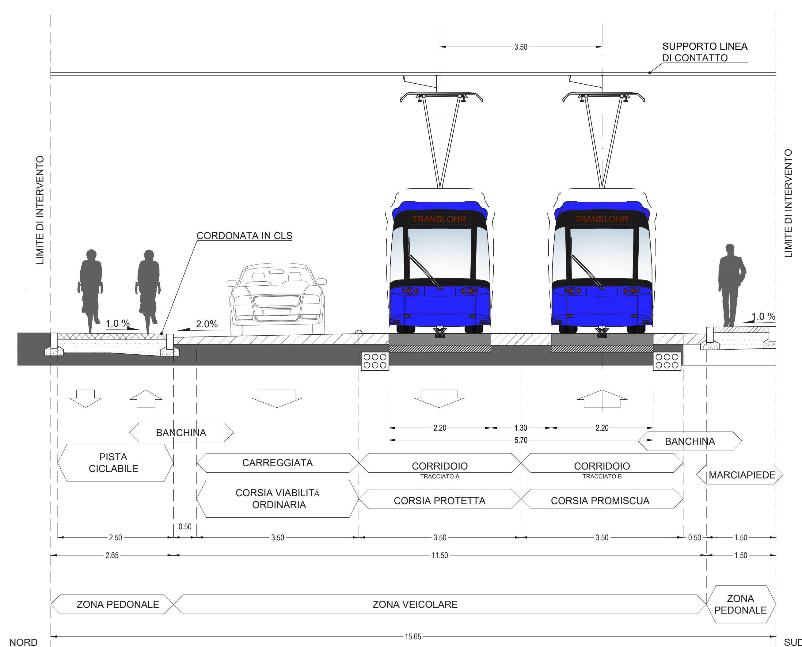
SEZIONE 9 SCALA 1:50
