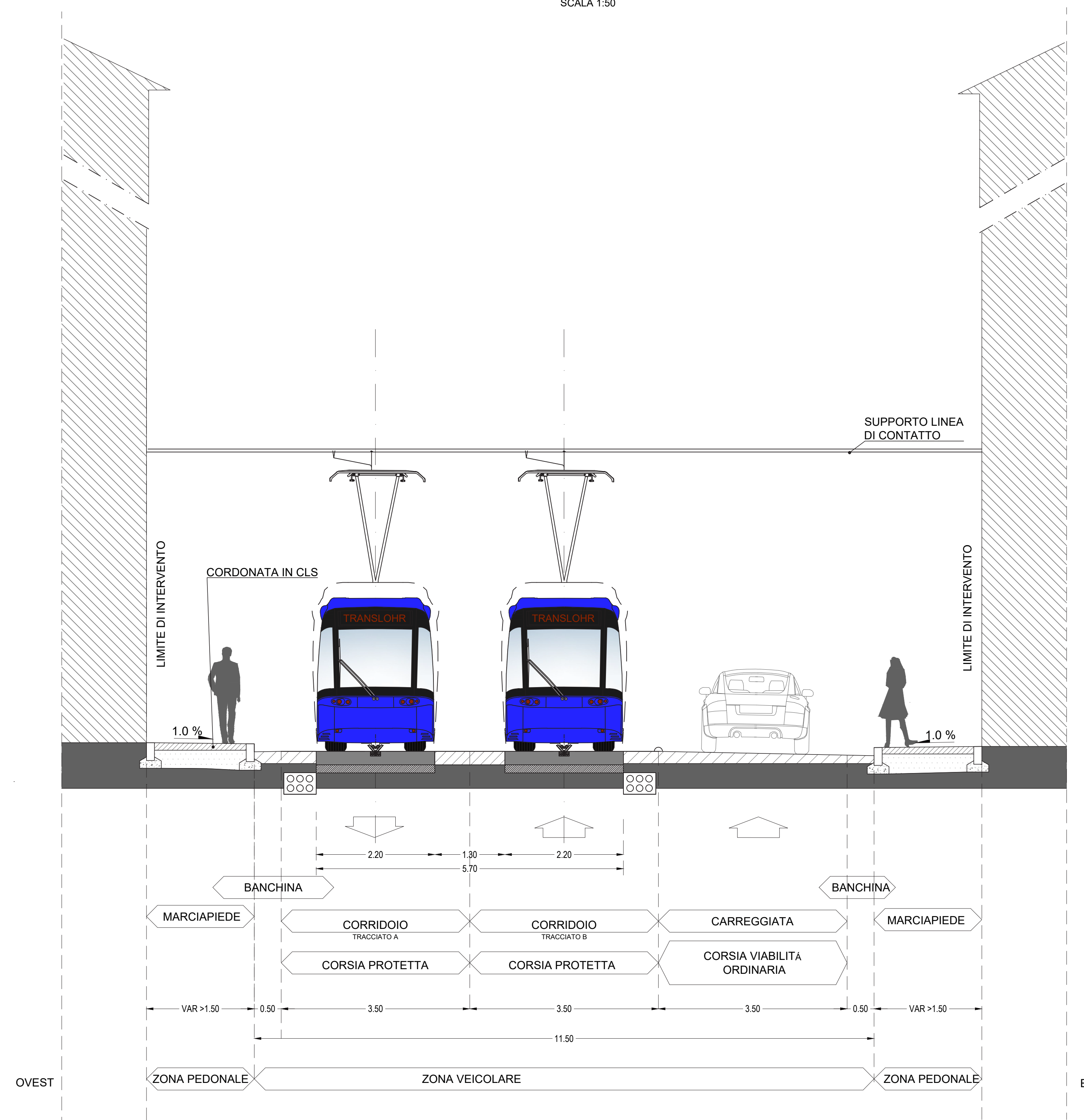
SEZIONE 6 SEZIONE TIPOLOGICA "CORSO GARIBALDI" SCALA 1:50
