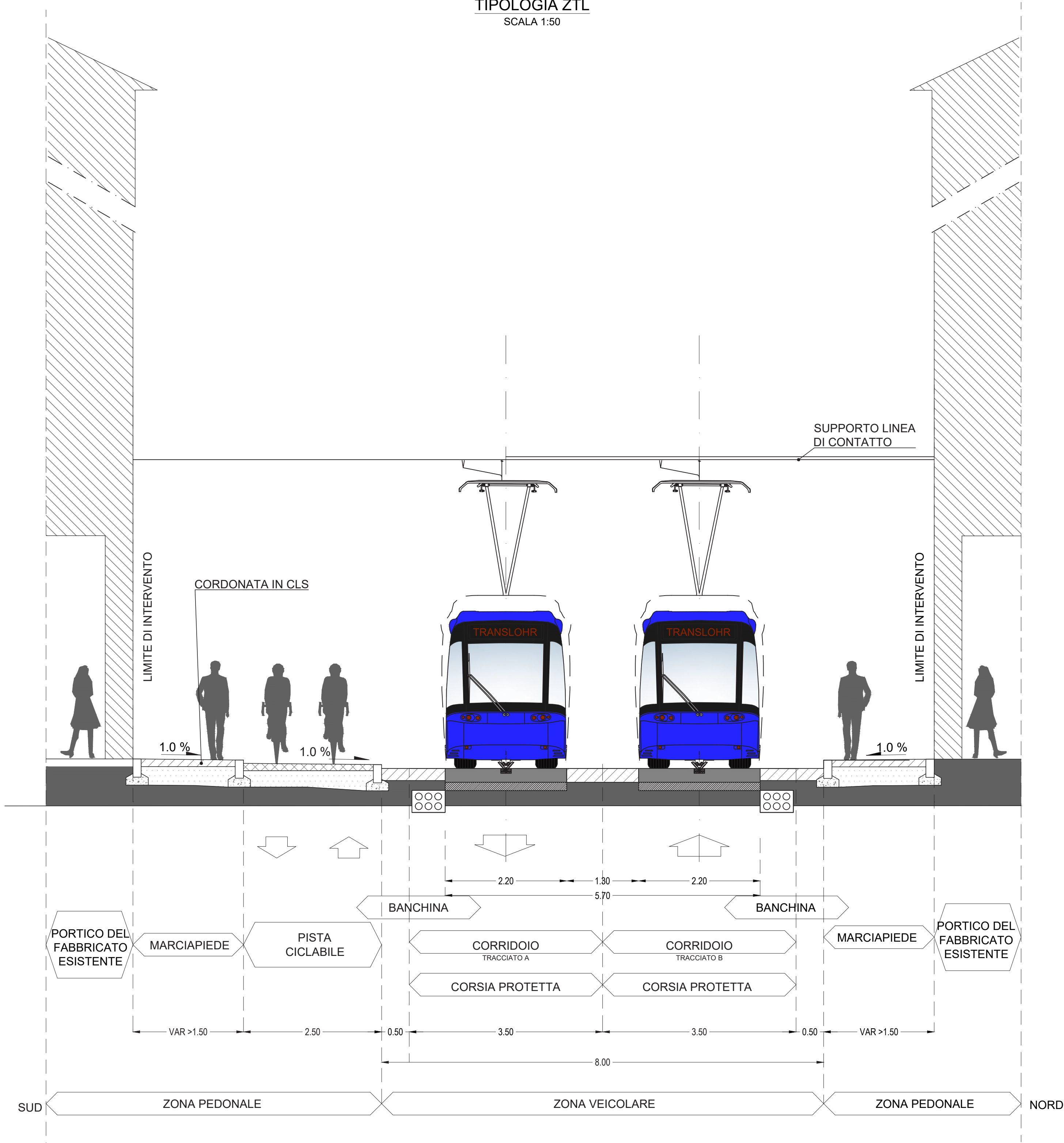
SEZIONE 5 TIPOLOGIA ZTL SCALA 1:50
