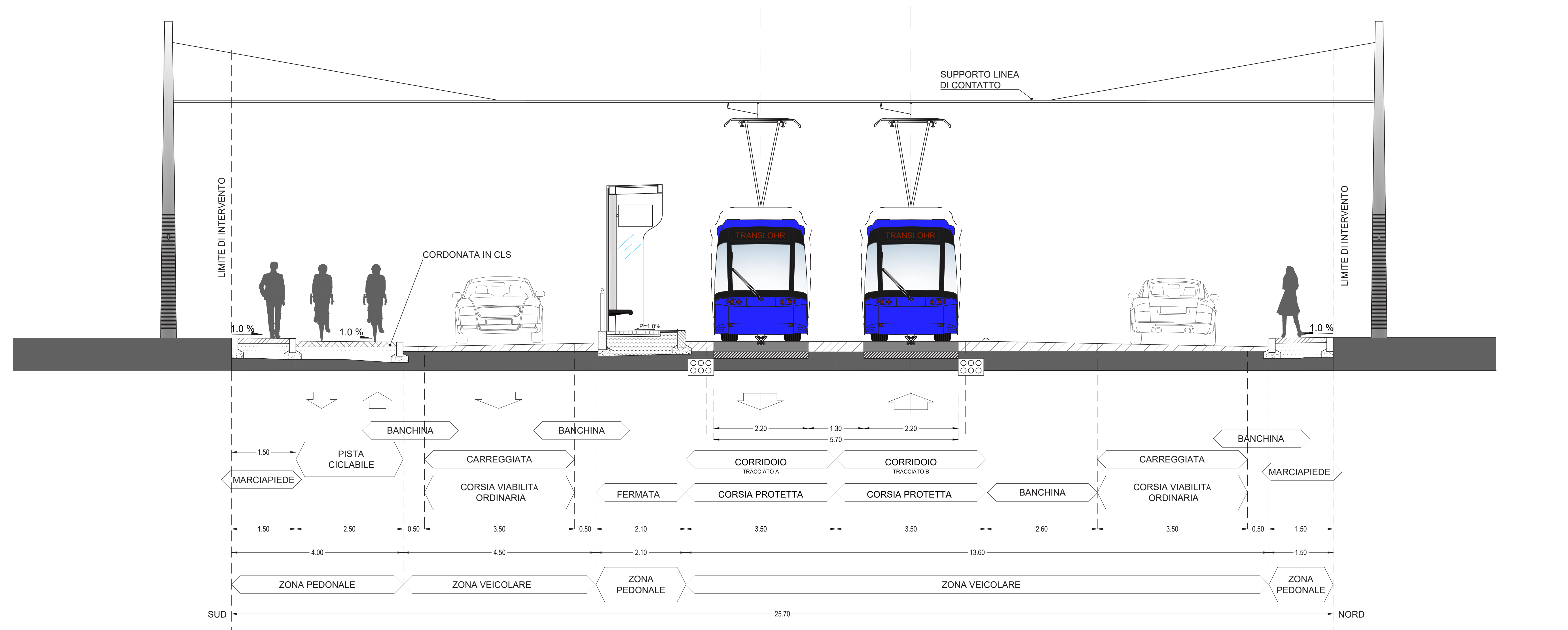
SEZIONE 2 SEZIONE TIPOLOGICA "FERMATA" SCALA 1:50
