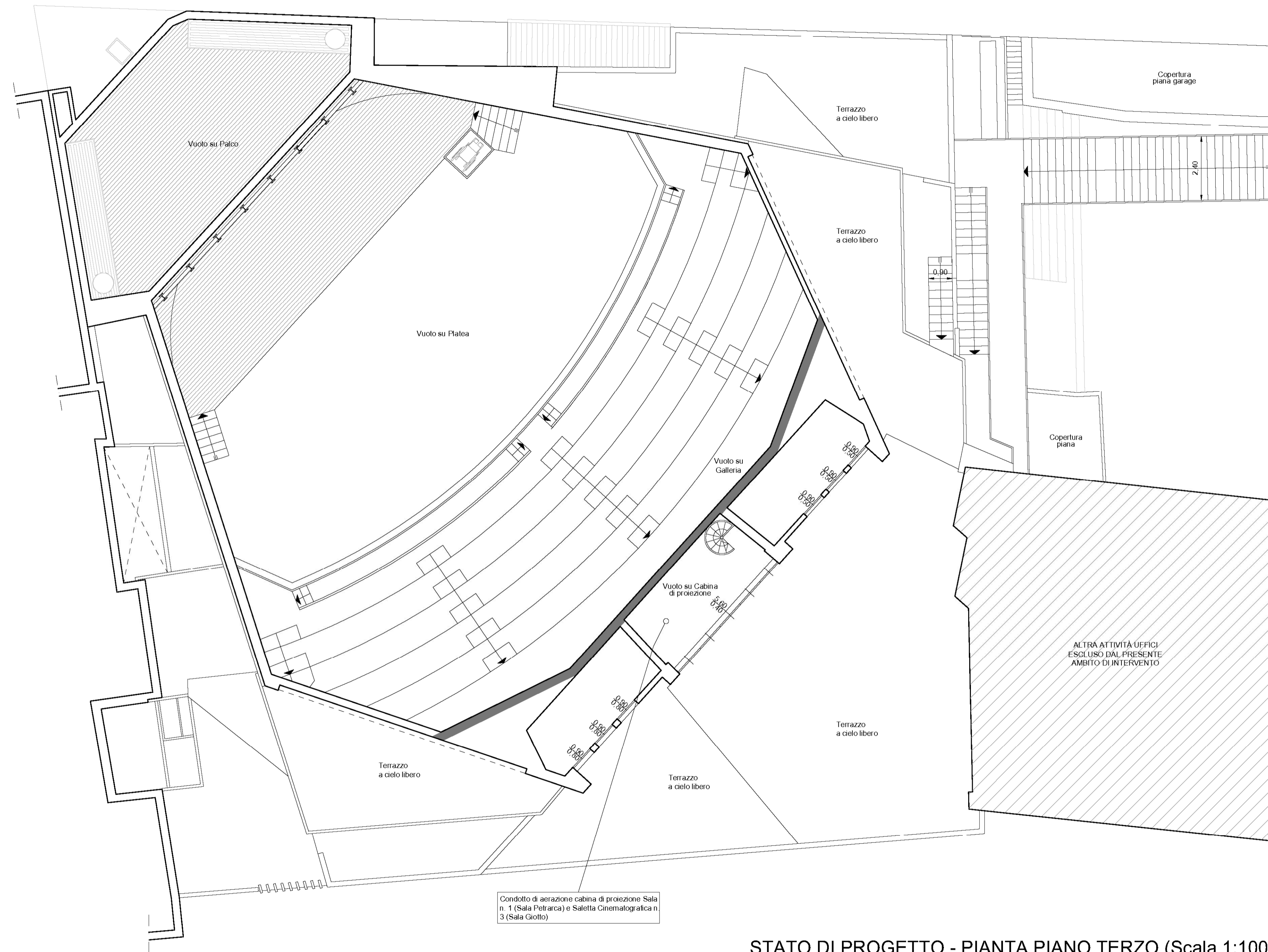
STATO DI PROGETTO - PIANTA PIANO TERZO (Scala 1:100)
