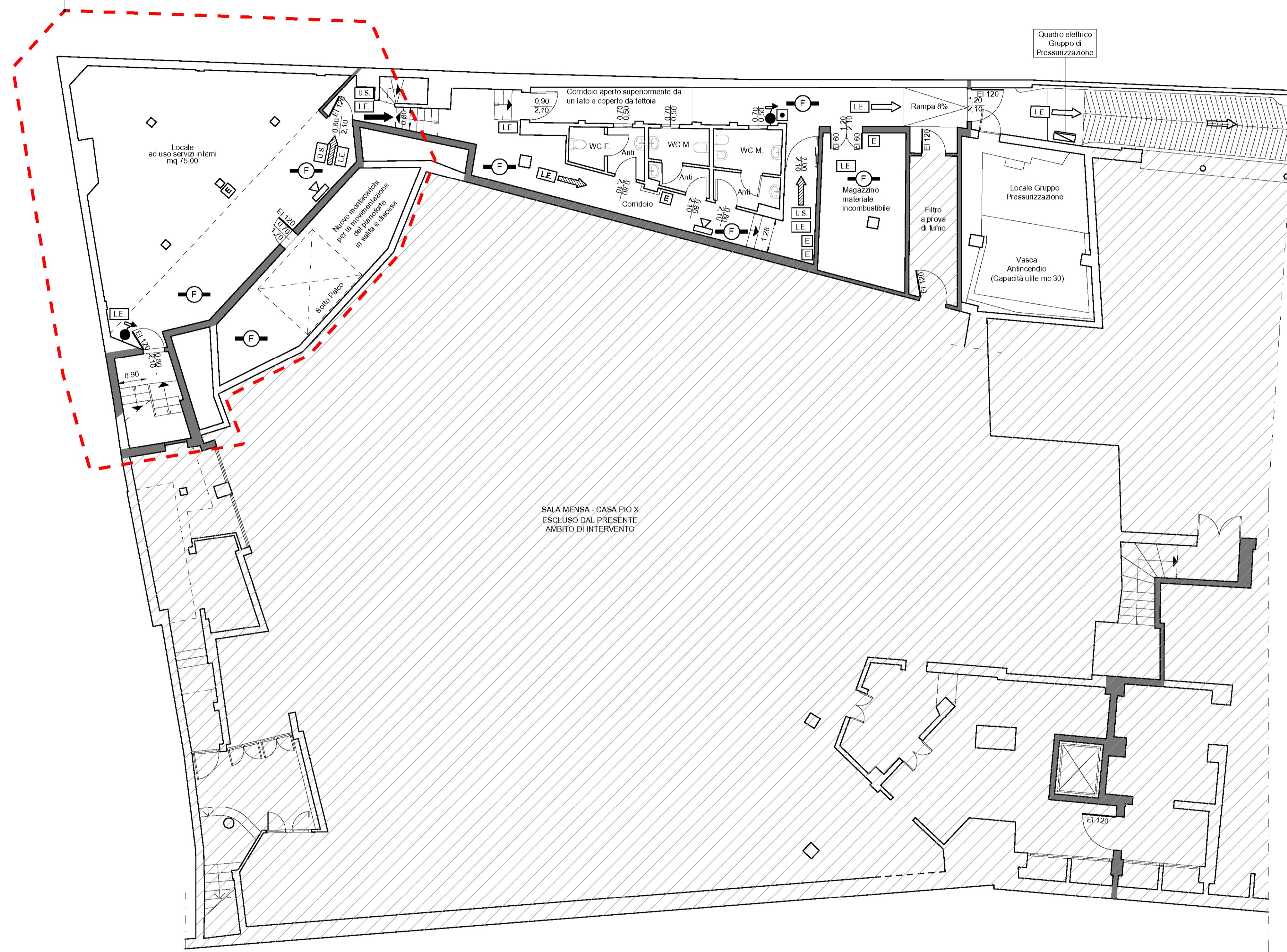
STATO DI PROGETTO - PIANTA PIANO INTERRATO (Scala 1:100)
