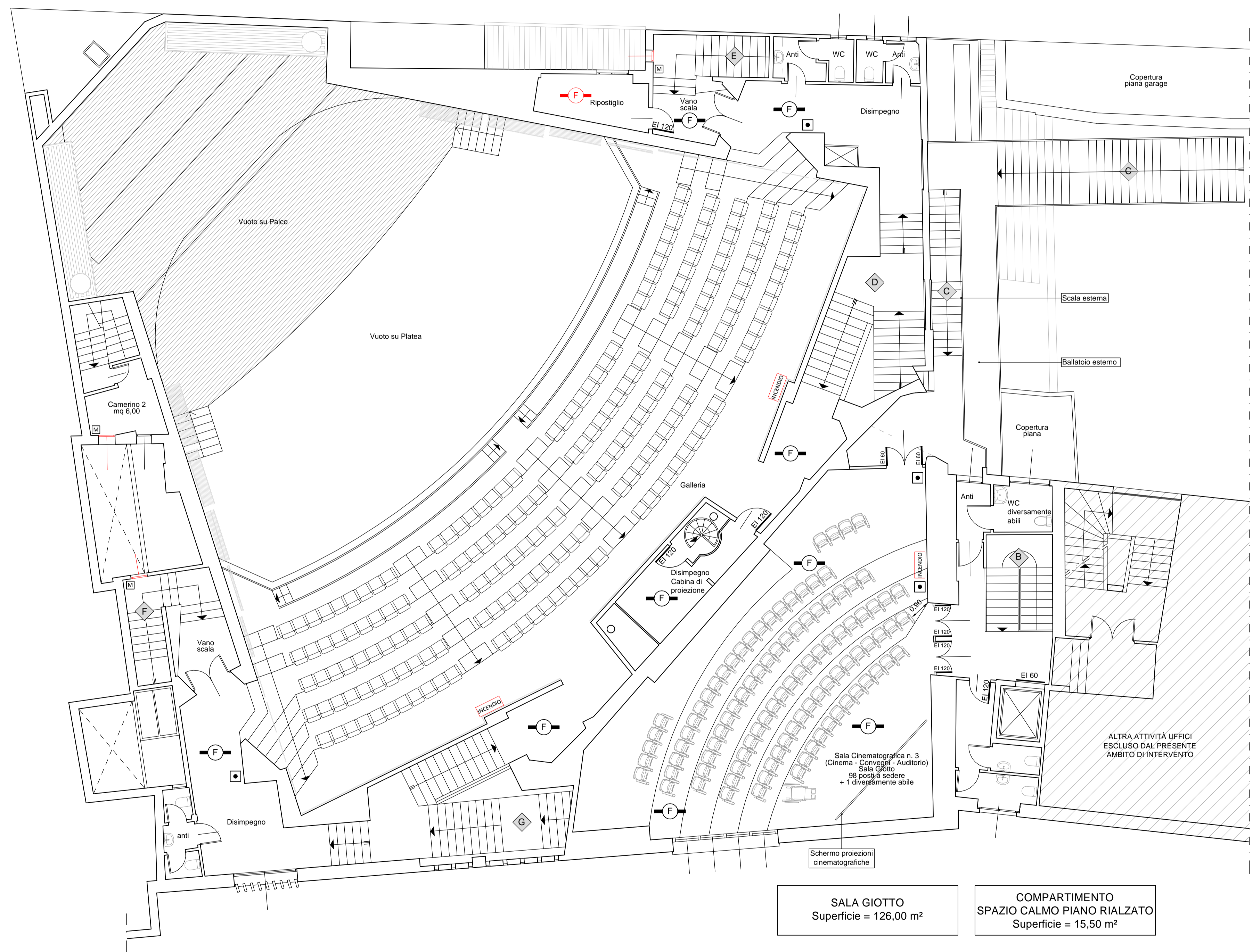
PIANTA PIANO PRIMO RIALZATO (Scala 1:100)
