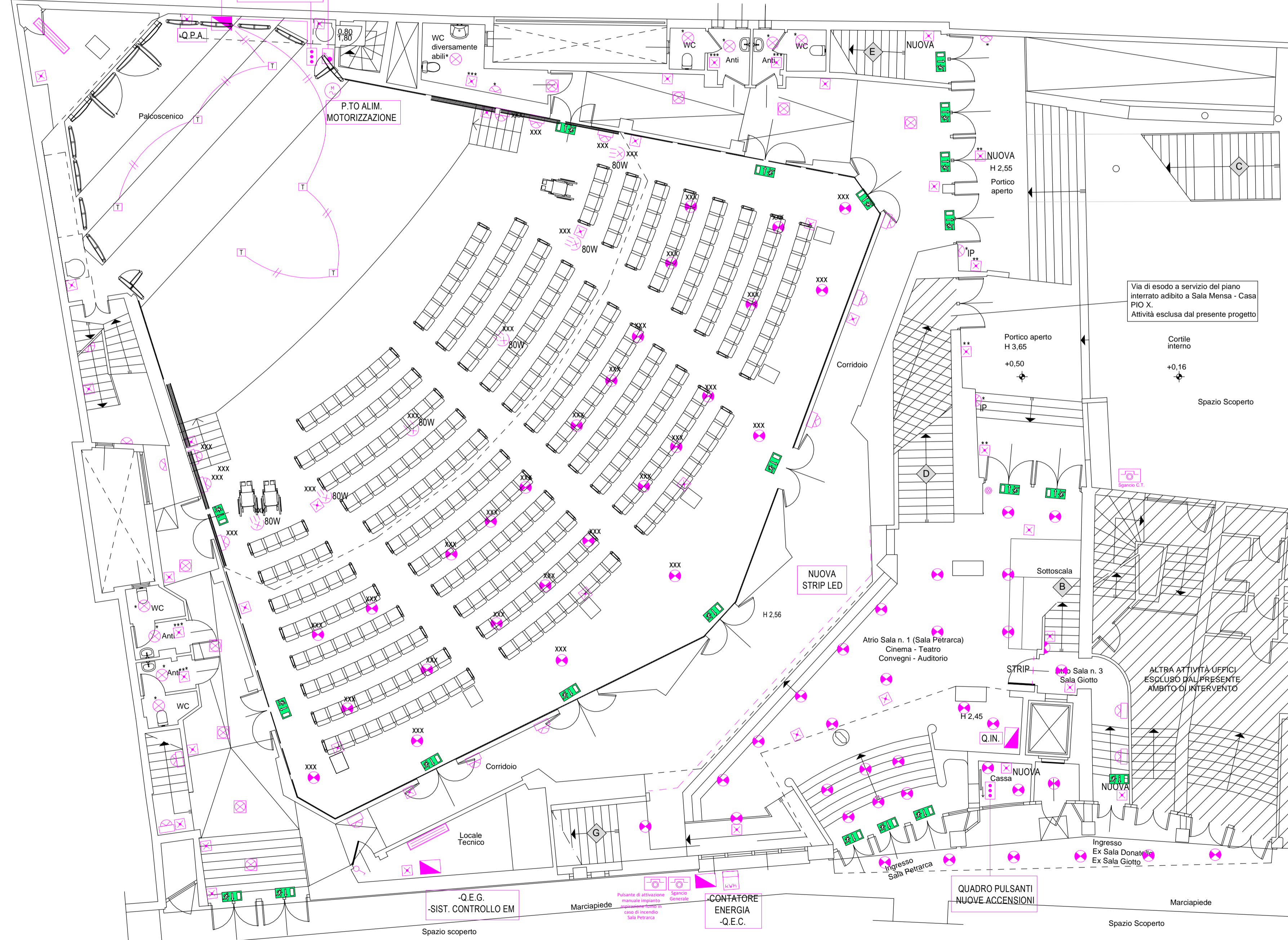
STATO DI PROGETTO - PIANTA PIANO TERRA (Scala 1:100)
