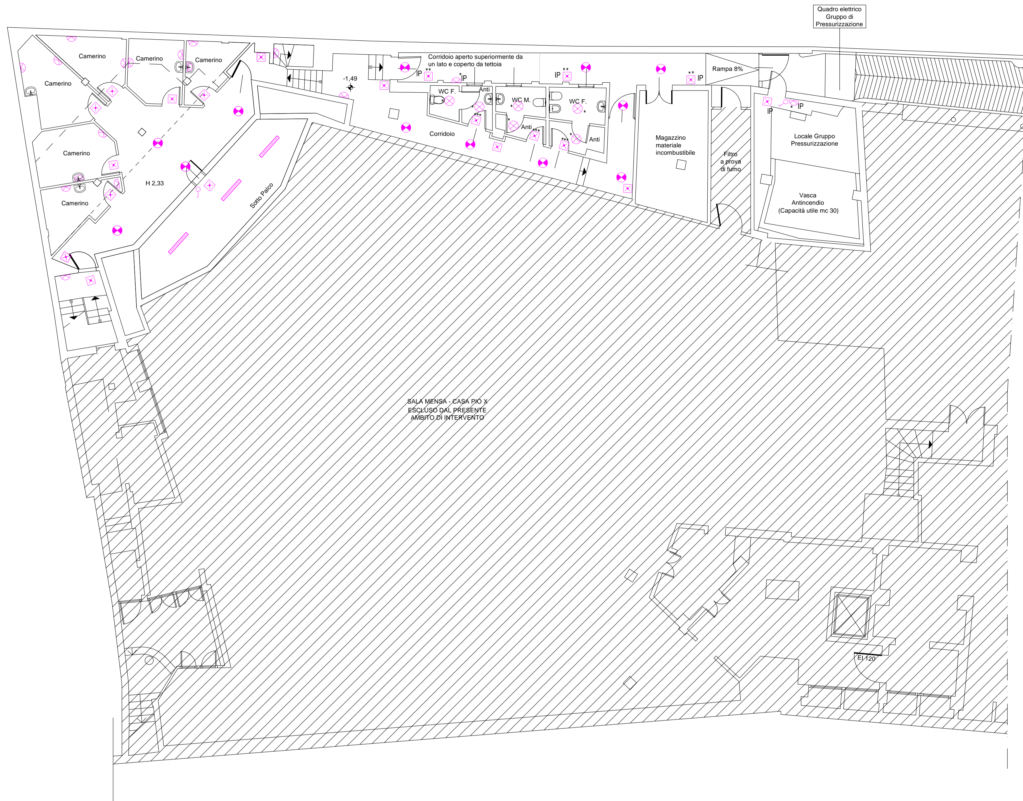
STATO DI PROGETTO - Pianta Piano Interrato (Sacla 1:100)
