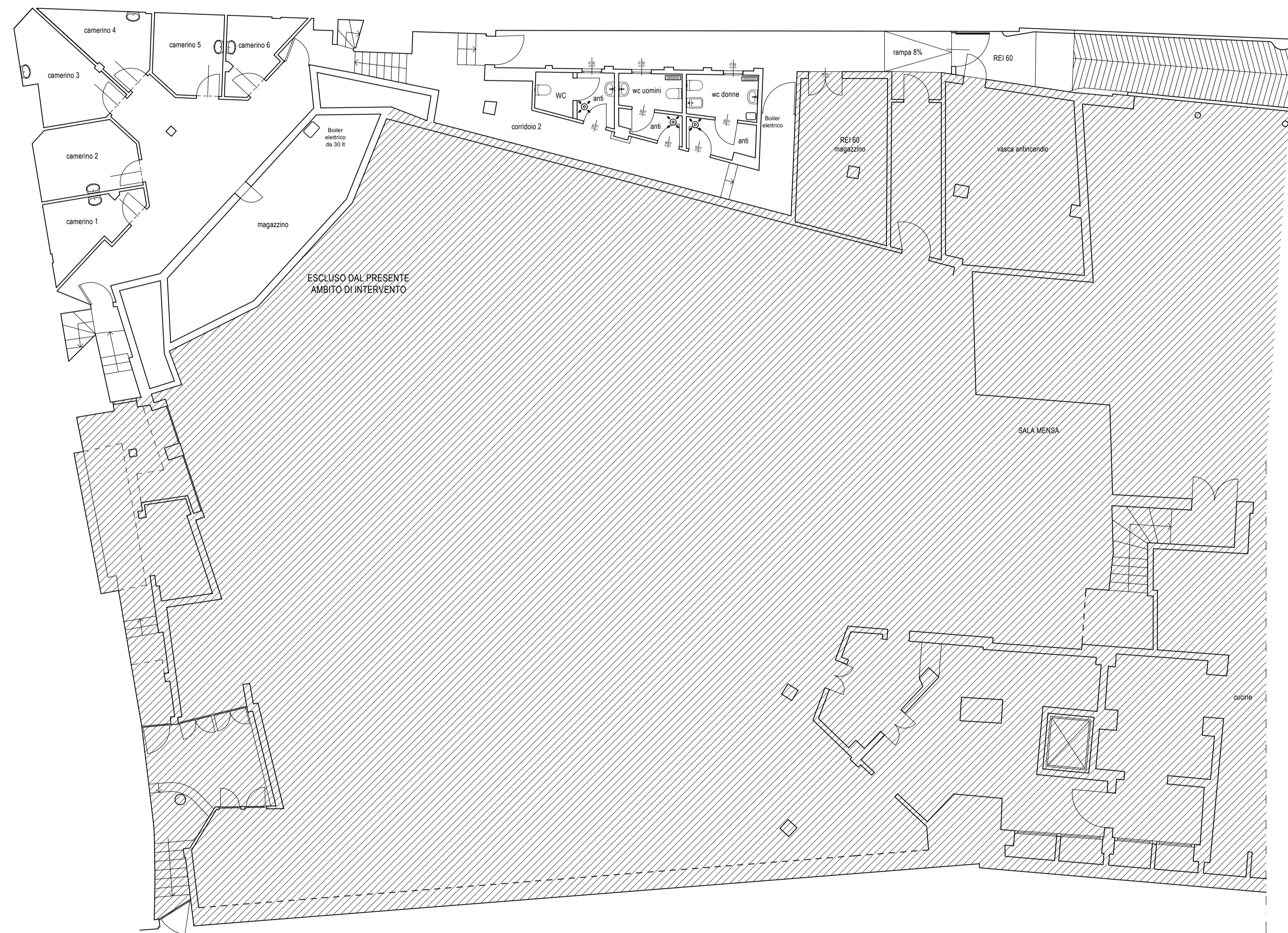
STATO DI PROGETTO PIANTA PIANO INTERRATO
