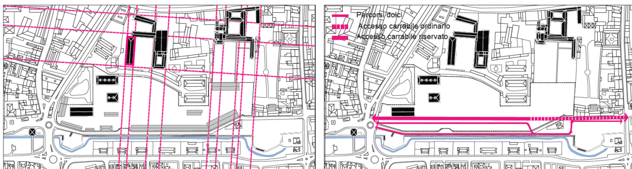
Figura 2. L'immagine esemplifica la relazione dell'area di progetto con i segni storici e con le tracce naturali del passato. Segni che il progetto riprende e reinterpreta per la definizione del nuovo assetto dell'area in coerenza con quanto indicato nel DOCFAP.
