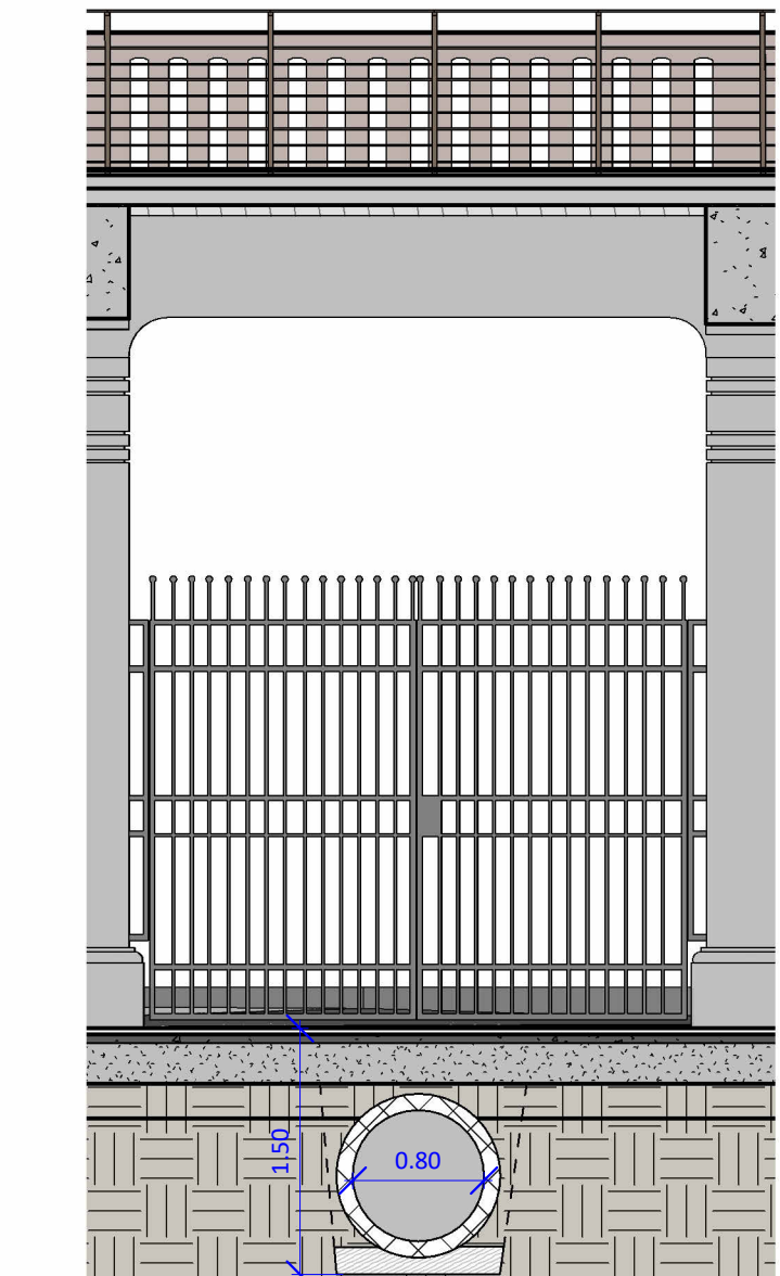
DETTAGLIO CUNICOLO SOTTOSERVIZI 1:50
