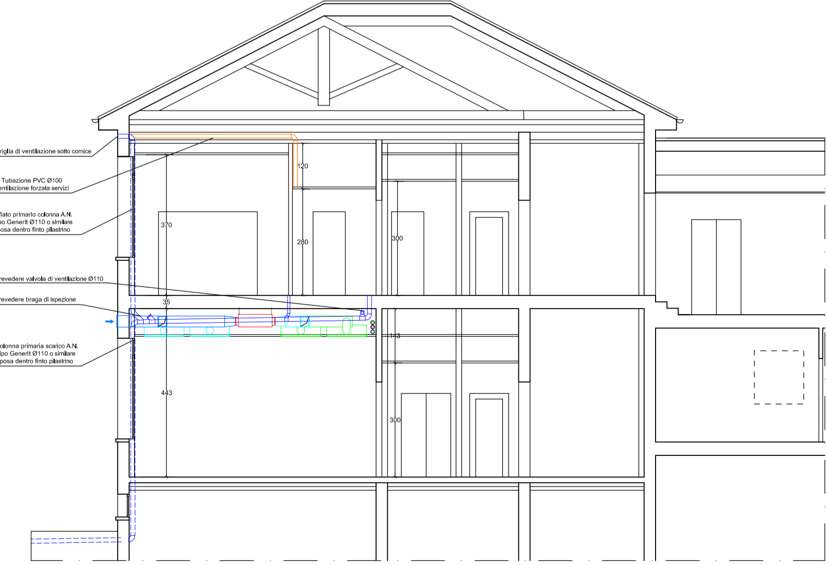
SEZIONE
