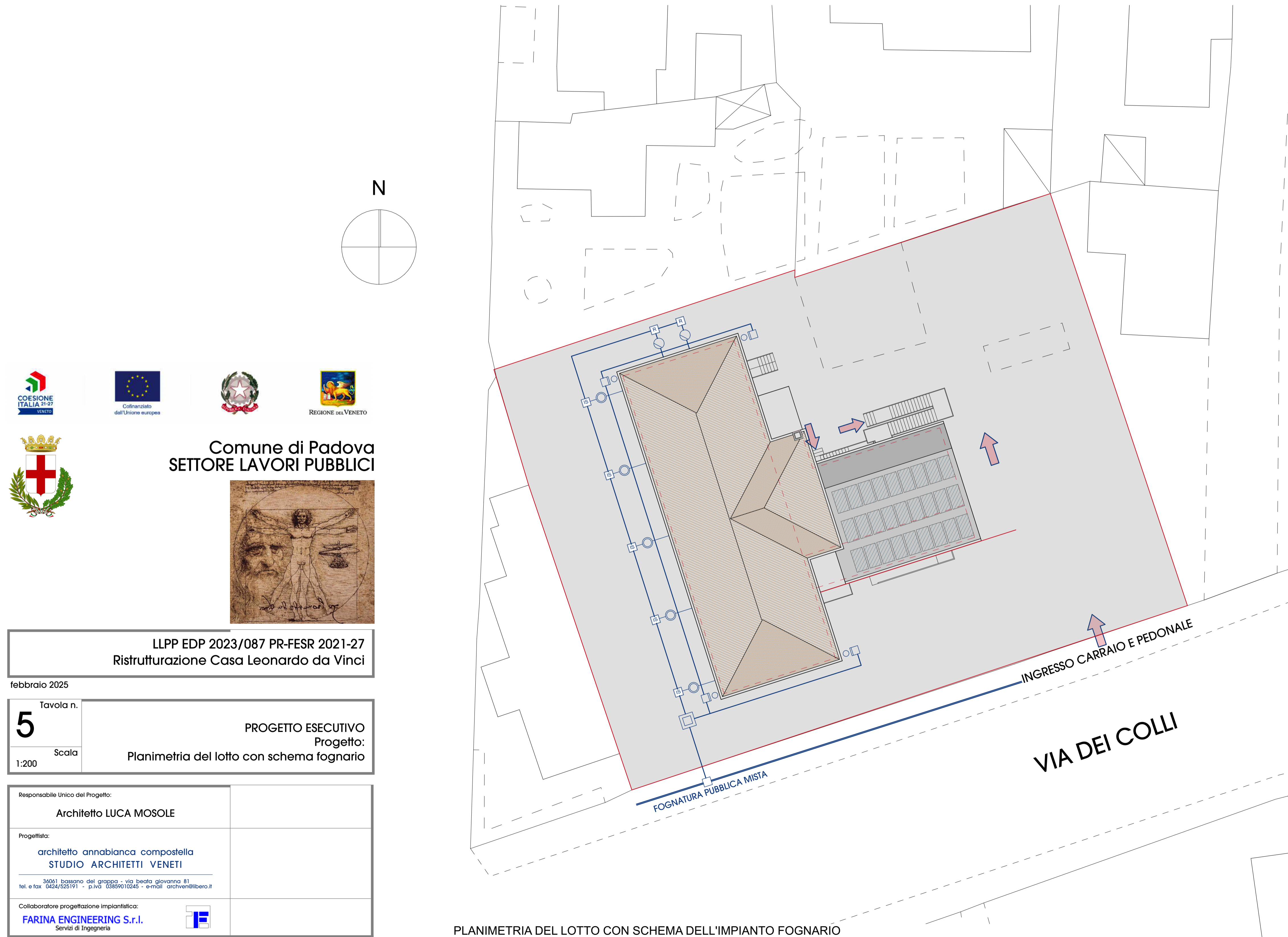
PLANIMETRIA DEL LOTTO CON SCHEMA DELL'IMPIANTO FOGNARIO
